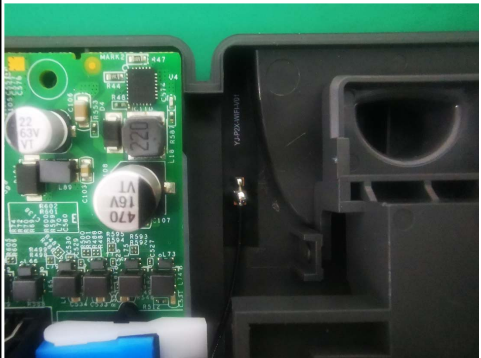
2.4G Antenna
