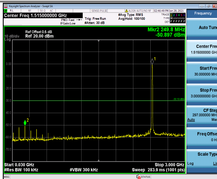
11B_Ant1_2437_30~3000
