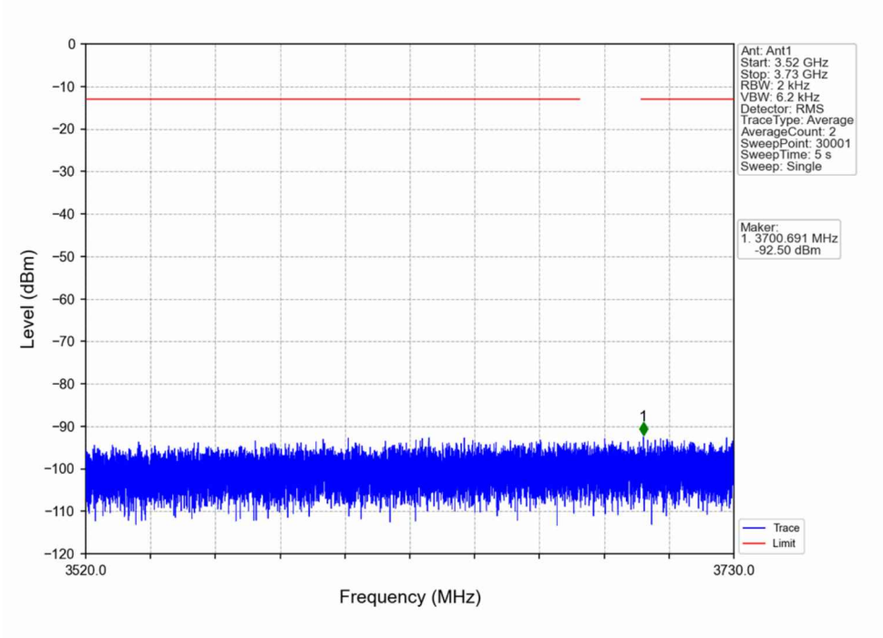
n48_30kHz_SISO_NTNV_20MHz_CP-OFDM QPSK_3690MHz_Inner_1RB_Right
