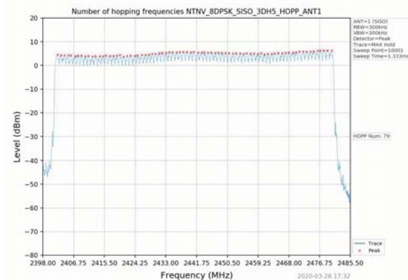
8DPSK_Hopping_3DH5_SISO_ANT1
