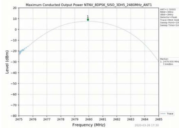
8DPSK_2480MHz_3DH5_SISO_ANT1
