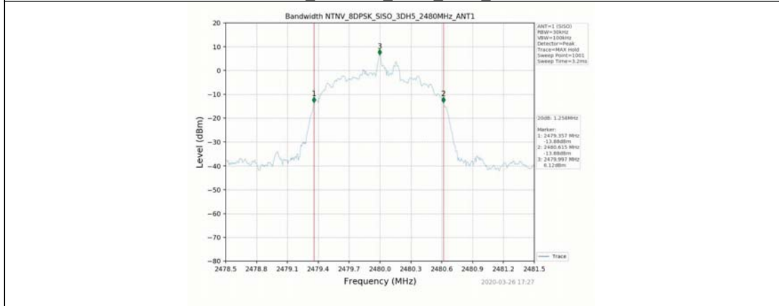
8DPSK_2480MHz_3DH5_SISO_ANT1
