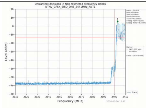
GFSK_Hopping_DH5_SISO_ANT1
