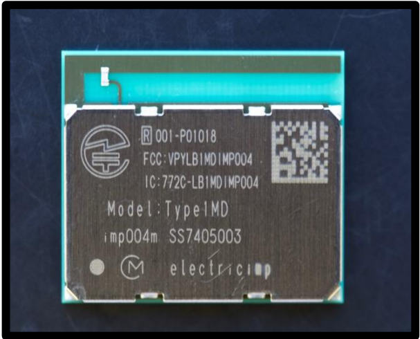
EUT Photo
