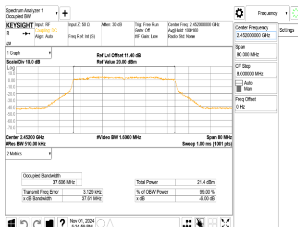
802.11ax 40MHz ChainB 2452MHz
