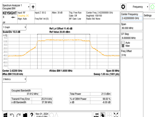
802.11ax 40MHz ChainB 2422MHz
