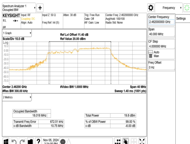
802.11be_20MHz_ChainB_2462MHz_106+26_MRU2
