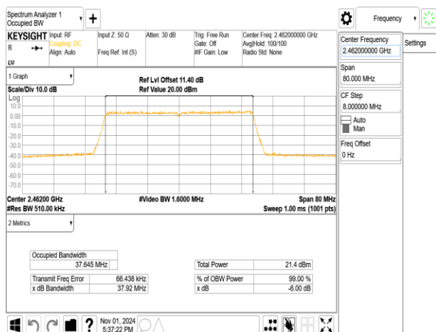
802.11ax 40MHz ChainA 2462MHz RU242 62
