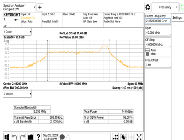
802.11be_20MHz_ChainA_2462MHz_RU52_40
