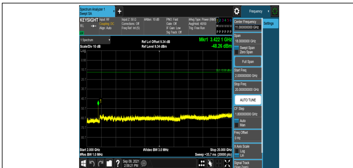
Band4-15MHz-QPSK-20025-1RB#0-Range5:2000~20000MHz
