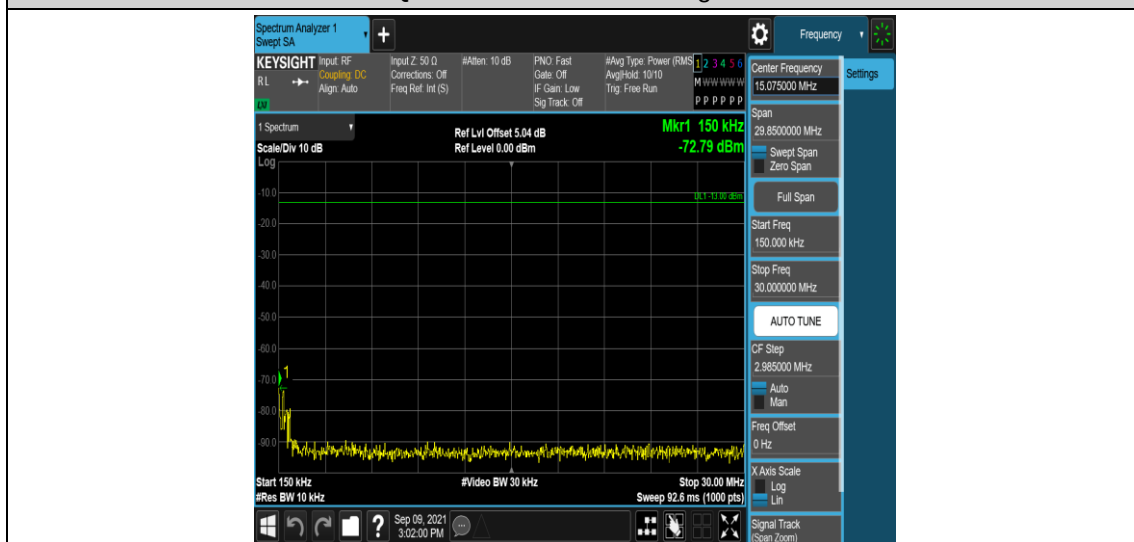
Band4-15MHz-QPSK-20325-1RB#0-Range2:0.15~30MHz
