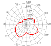
2500.000MHz E2
