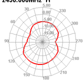
2450.000MHz H
