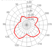
2500.000MHz H
