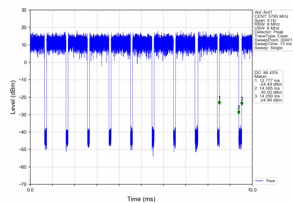
802.11n(HT20)_MCH_5785MHz_Ant1_NTNV
