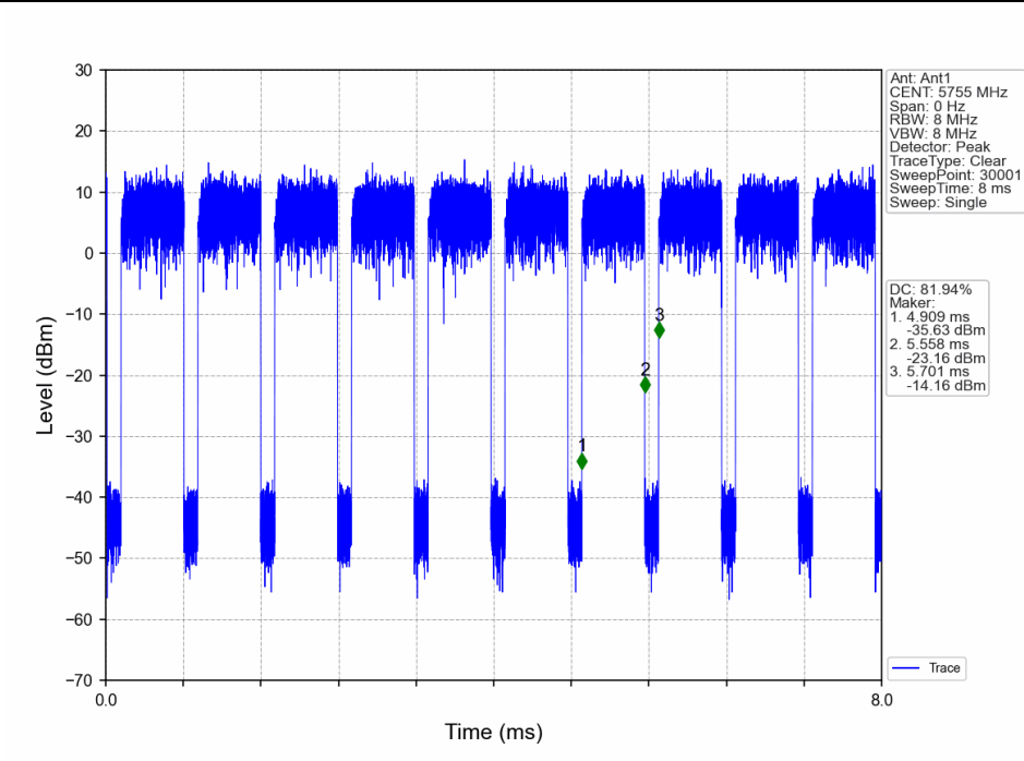
802.11n(HT40)_LCH_5755MHz_Ant1_NTNV
