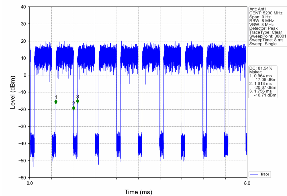
802.11n(HT40)_HCH_5230MHz_Ant1_NTNV
