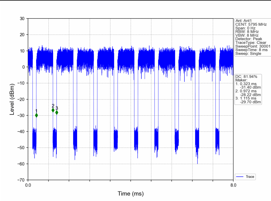
802.11n(HT40)_HCH_5795MHz_Ant1_NTNV
