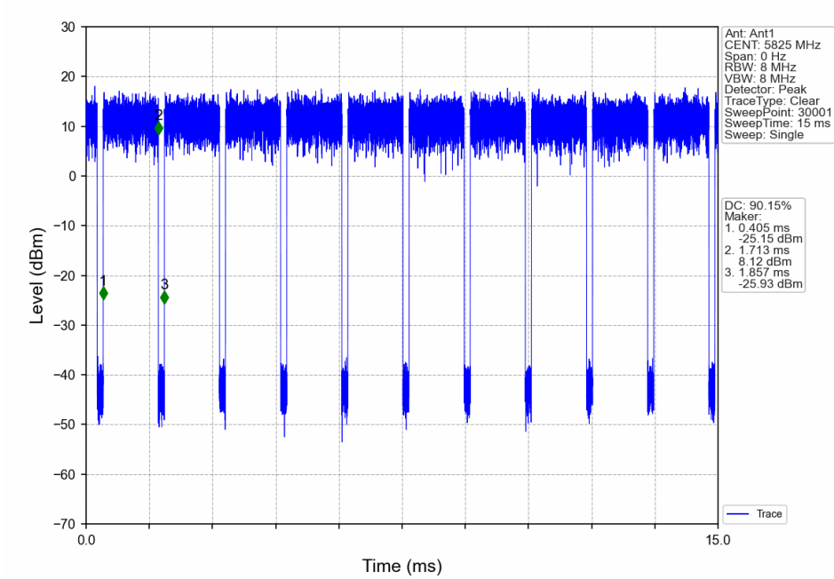
802.11n(HT20)_HCH_5825MHz_Ant1_NTNV
