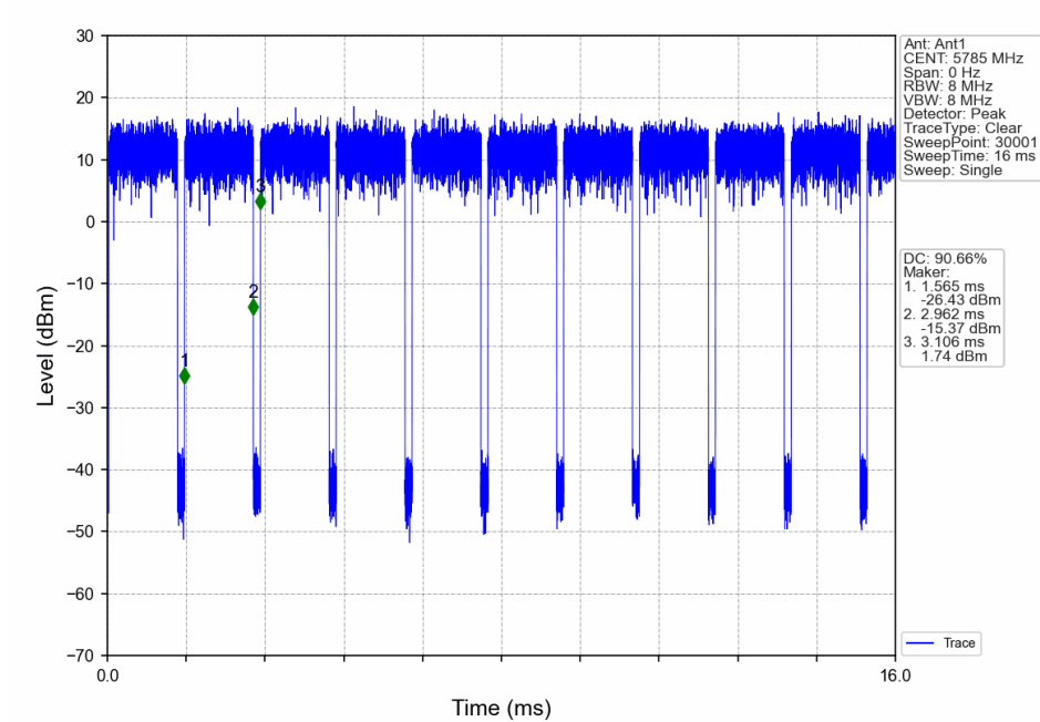
802.11a_MCH_5785MHz_Ant1_NTNV
