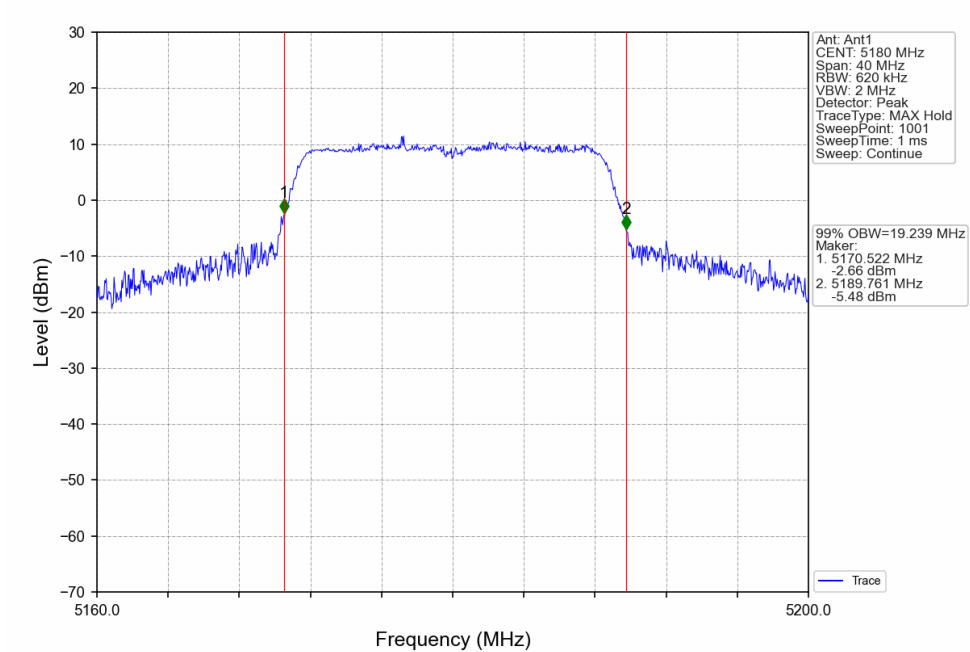
802.11n(HT20)_LCH_5180MHz_Ant1_NTNV
