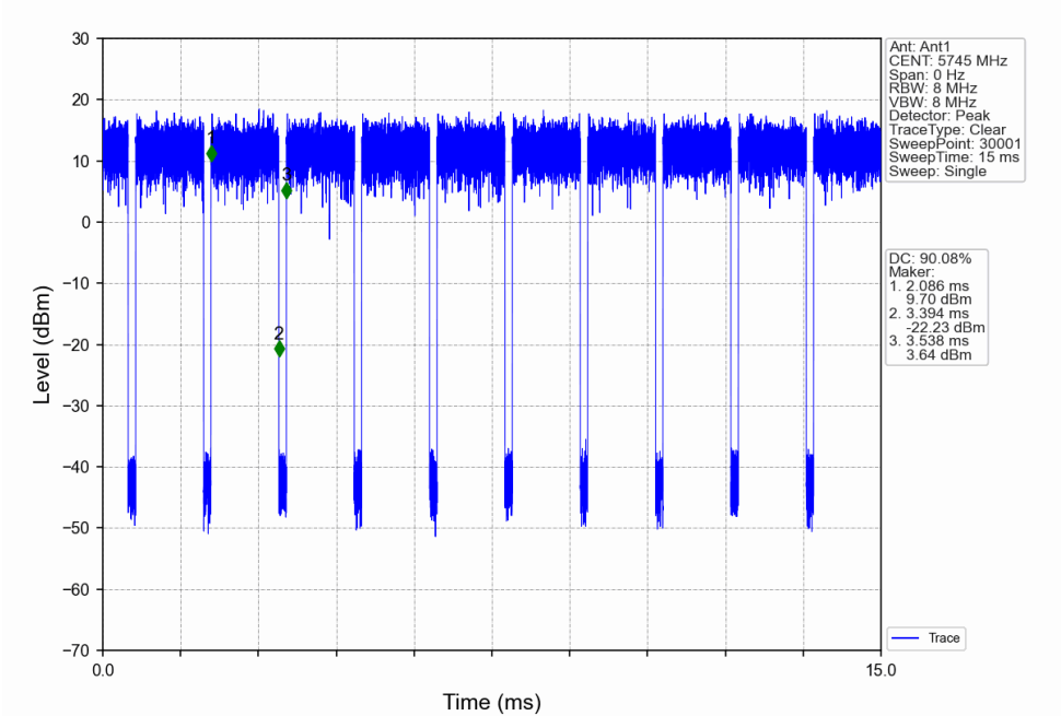
802.11n(HT20)_LCH_5745MHz_Ant1_NTNV
