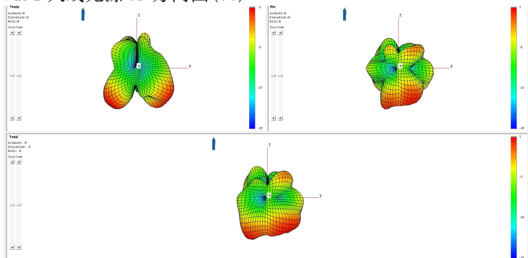
WIFI 天线无源 3D 方向图(5G)
