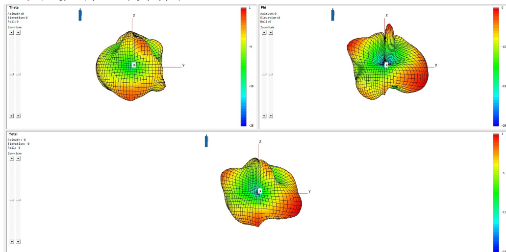
BT 天线无源 3D 方向图
