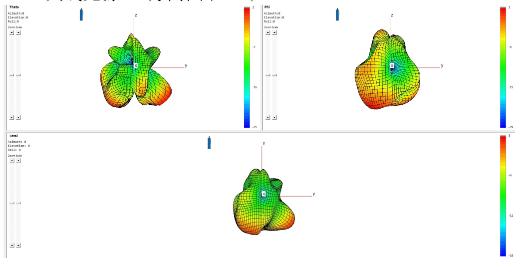
WIFI 天线无源 3D 方向图(2.4G)
