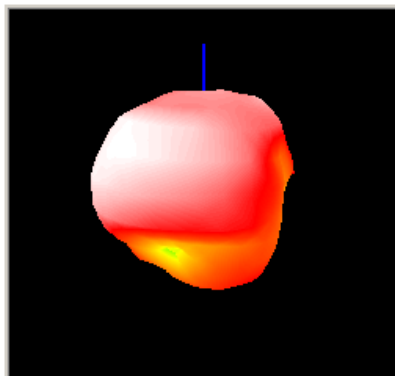
2.5GHz
