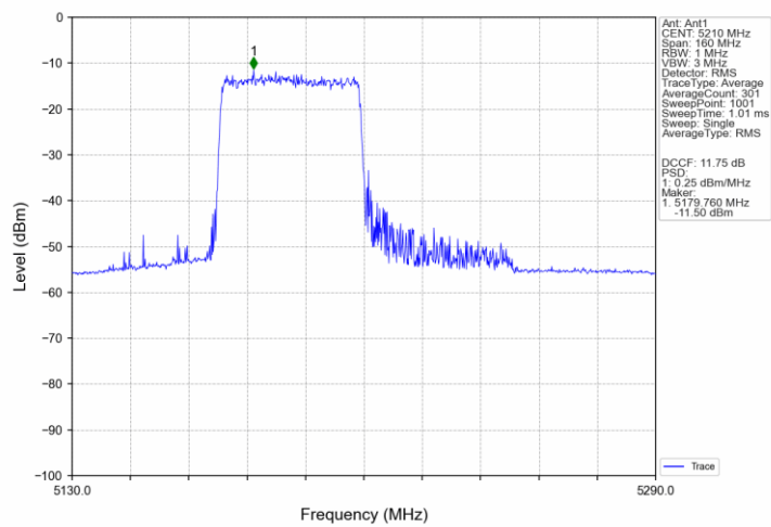
802.11ax(HEW80) MCH 5210MHz RU996 Left Ant1 NTN
