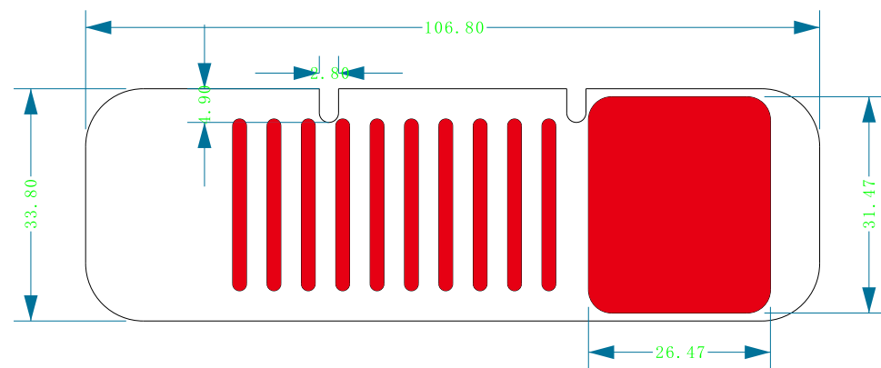
上壳贴纸 upper shell sticker
