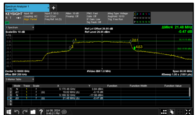
Figure 333 - 802.11ax HE20 SU Maximum 99% OBW
