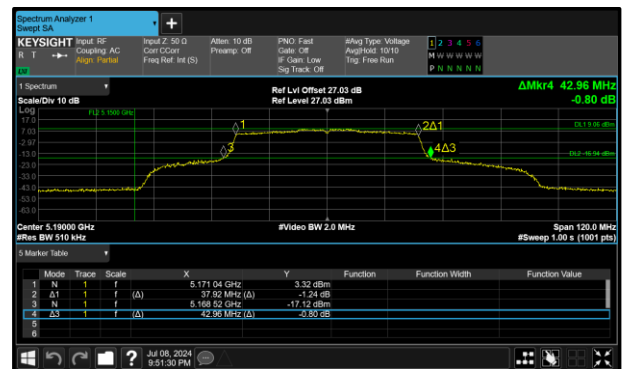
Figure 335 - 802.11ax HE40 SU Maximum 99% OBW
