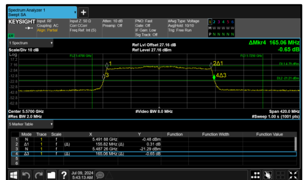
Figure 339 - 802.11ax HE160 SU Maximum 99% OBW
