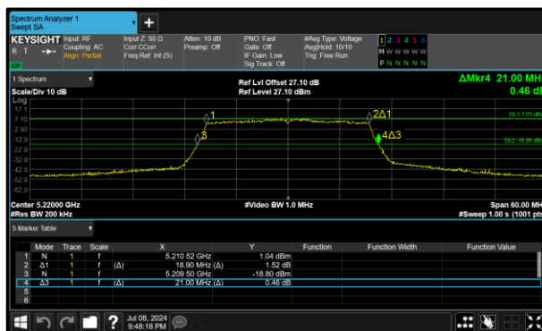
Figure 332 - 802.11ax HE20 SU Minimum 99% OBW
