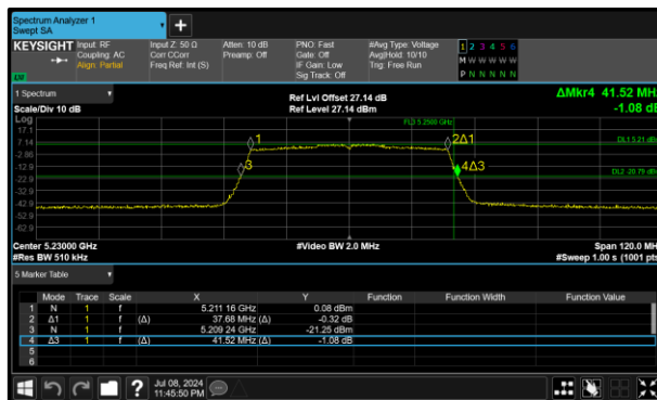
Figure 334 - 802.11ax HE40 SU Minimum 99% OBW
