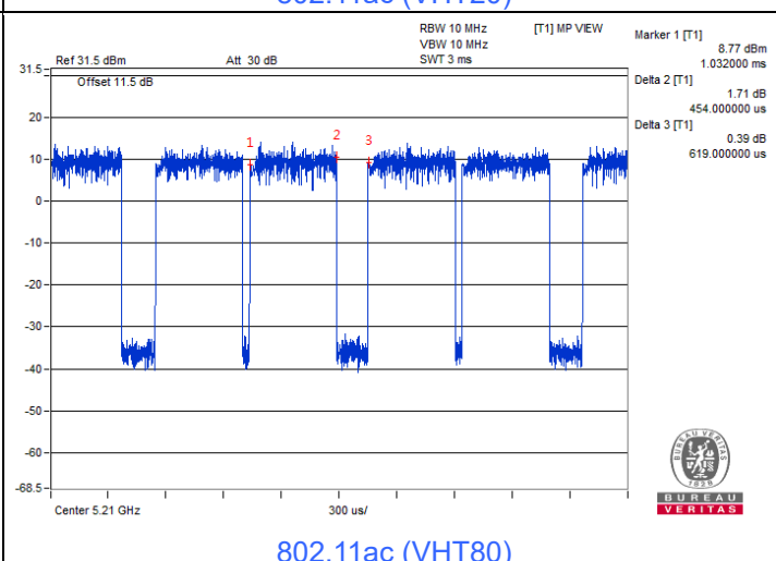
802.11ac (VHT80)
