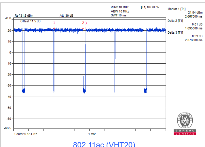
802.11ac (VHT20)
