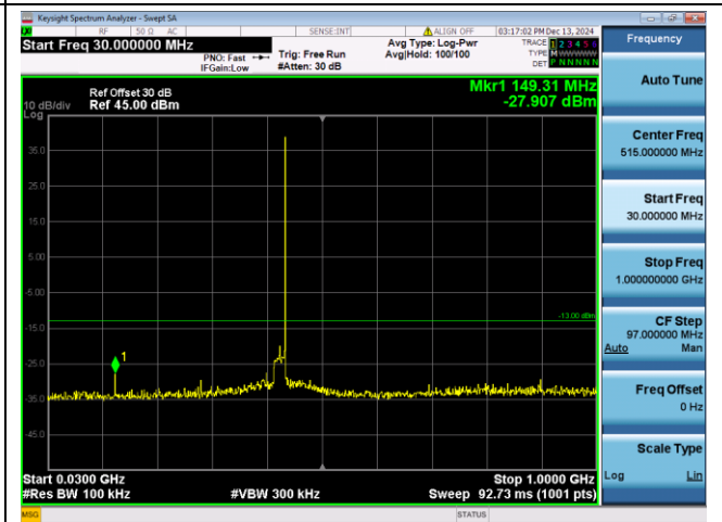
30MHz-1000MHz
