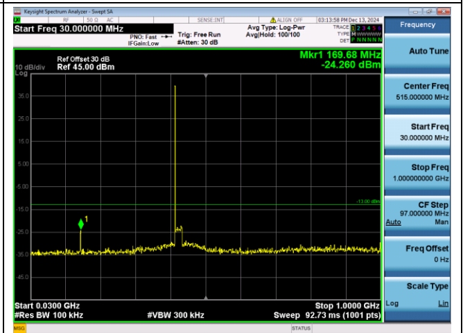
30MHz-1000MHz
