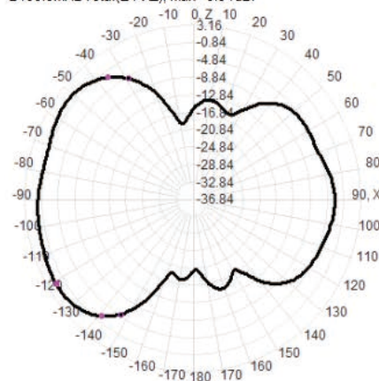
2400.0MHz Total(E1-XZ), Max= 0.94dBi
