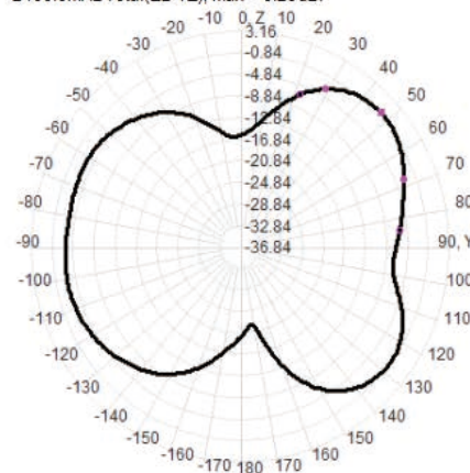
2400.0MHz Total(E2-YZ), Max= -0.29dBi
