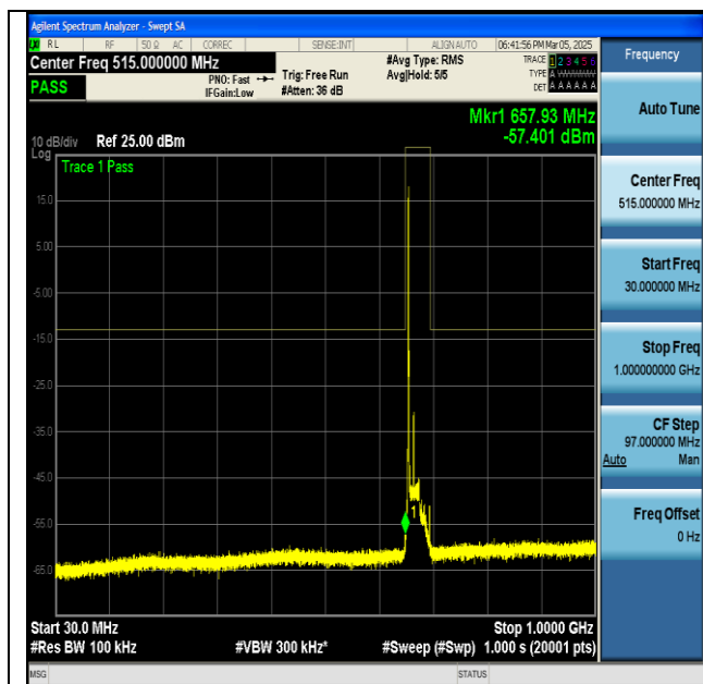
NTNV-n71-PC3-15-20-L-CP-QPSK-Edge_1RB_Left-30-1000-PASS
