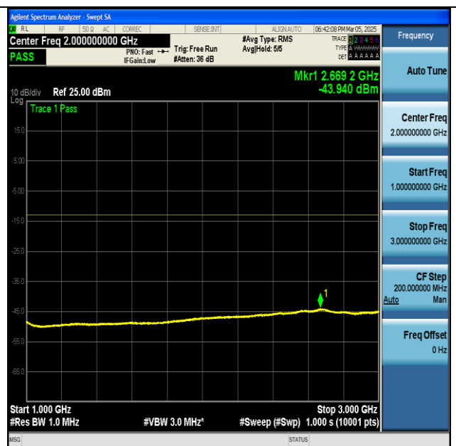
NTNV-n71-PC3-15-20-L-CP-QPSK-Edge_1RB_Left-1000-3000-PASS
