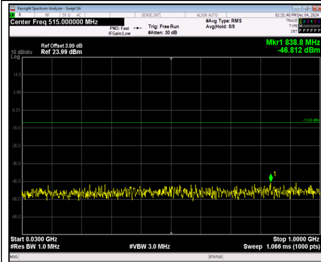
Band4-20MHz-QPSK-20300-1RB#0-Range1:30~100 0MHz
