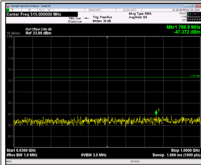
Band4-20MHz-QPSK-20175-1RB#0-Range1:30~100 0MHz
