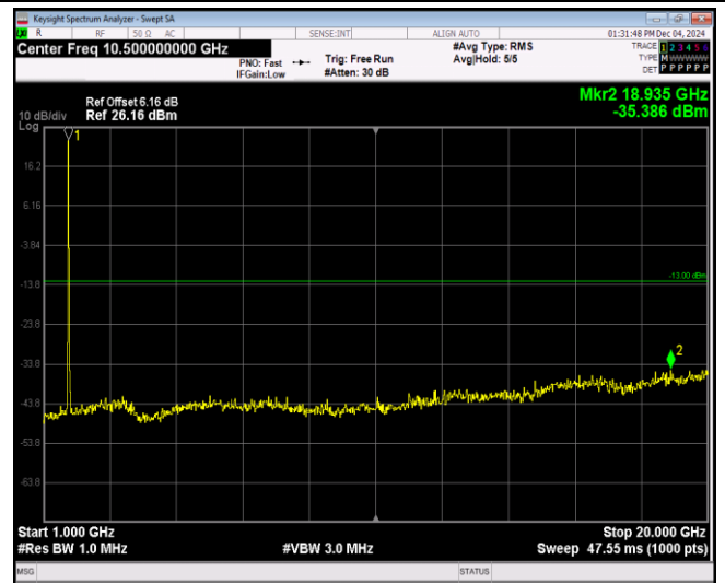
Band4-20MHz-QPSK-20300-1RB#0-Range2:1000~2 0000MHz
