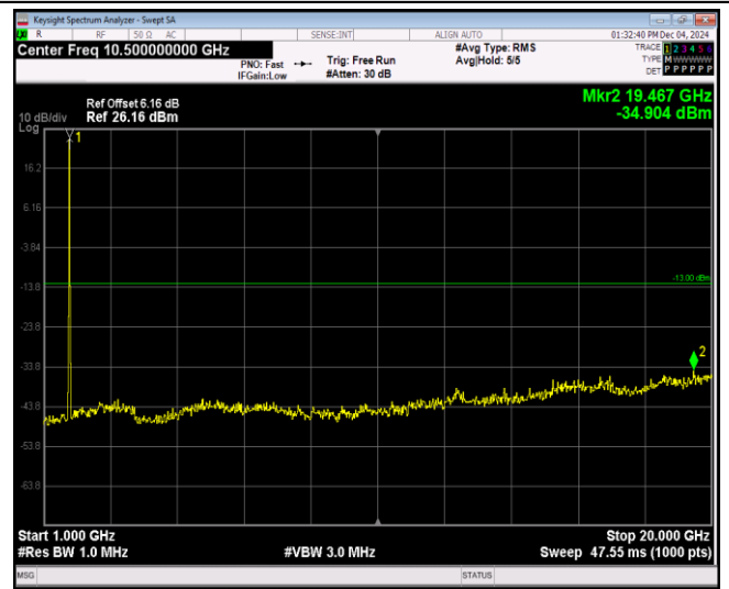
Band4-20MHz-QPSK-20300-1RB#0-Range2:1000~2 0000MHz
