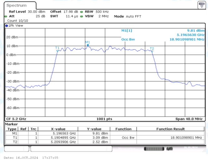
11AX20MIMO-Ant2-5200
