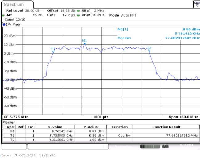
11AC80MIMO-Ant1-5775
