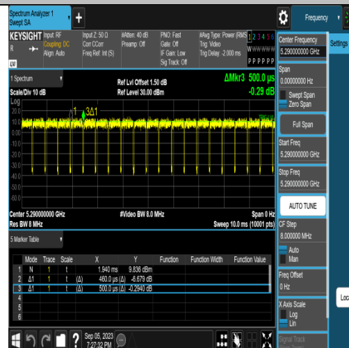
NTNV-11AC80SISO-Ant1-5290
