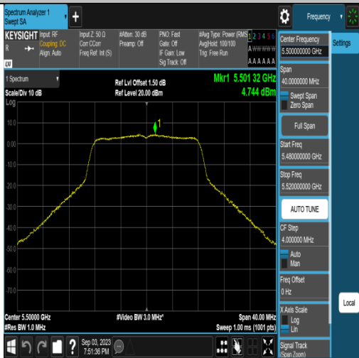
11A-Ant1-5500
