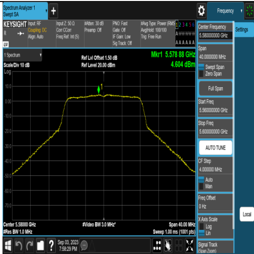
11A-Ant1-5580
