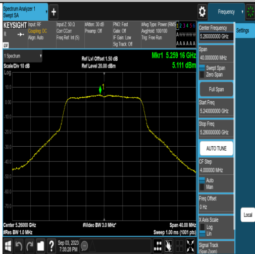
11A-Ant1-5260
