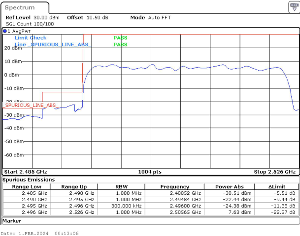
30MHz_30kHz_2511MHz_DFT-s-OFDM QPSK_RB75@0&-30.51 dBm
