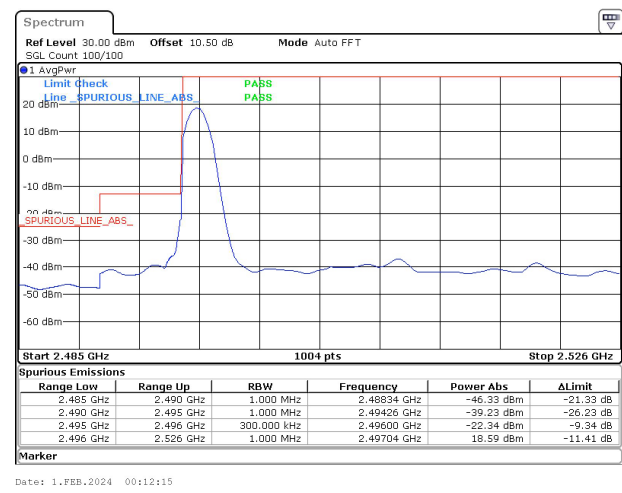
30MHz_30kHz_2511MHz_DFT-s-OFDM QPSK_RB1@0&-22.34 dBm
