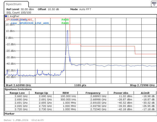
30MHz_30kHz_2674.98MHz_DFT-s-OFDM QPSK_RB1@77&-42.18 dBm
