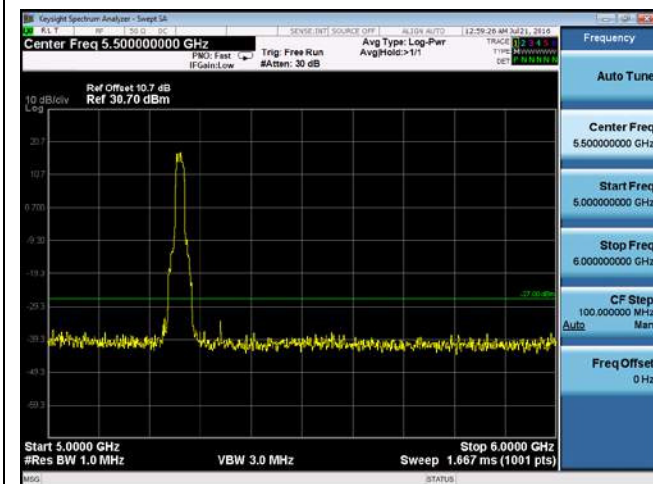
CUE-802.11a-5260-chain3(5GHz-6GHz)
