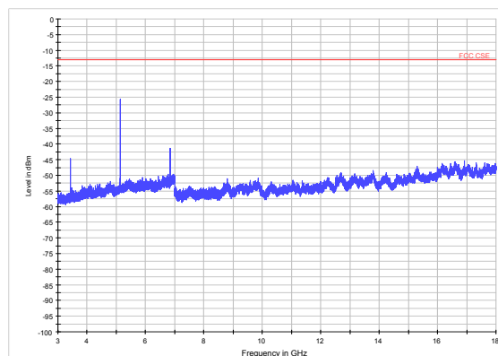
LTE Band 4 5MHz CH-Middle 3GHz~18GHz
