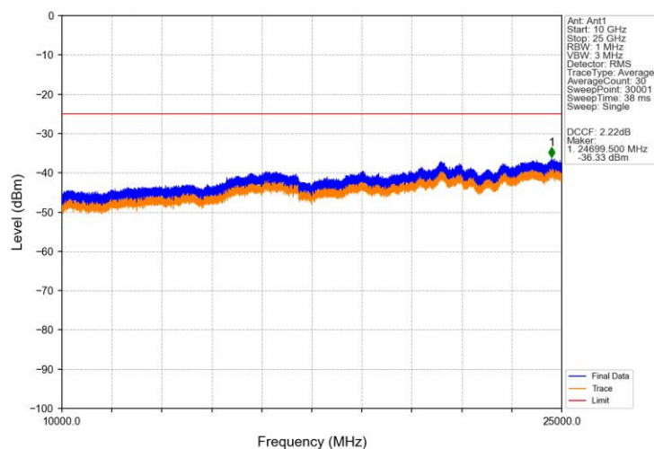
Band41_5MHz_QPSK_MCH_2593MHz_RB_1_0_NTNV
