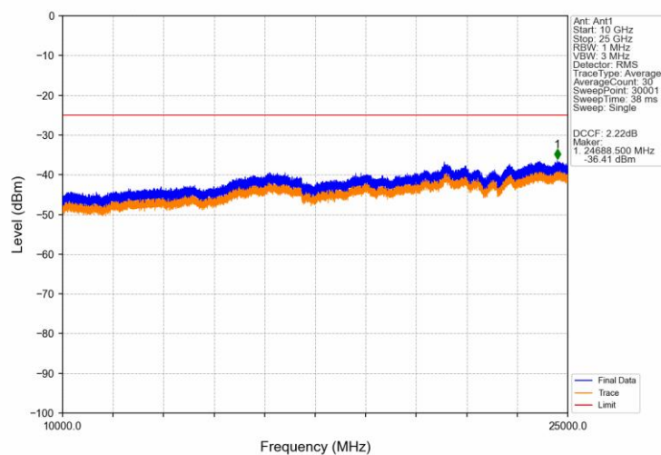
Band41_5MHz_QPSK_LCH_2498.5MHz_RB_1_0_NTNV
