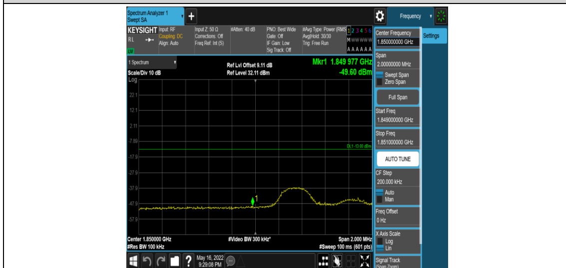
Band2-5MHz-QPSK-18625-1RB#24
