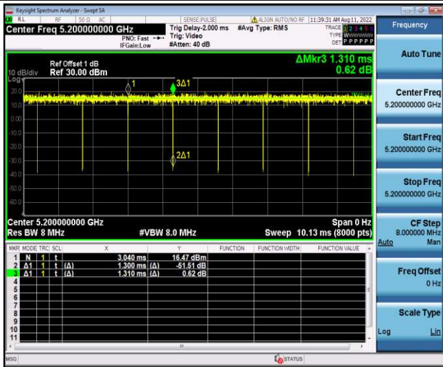
11N20SISO_Ant1_5200
