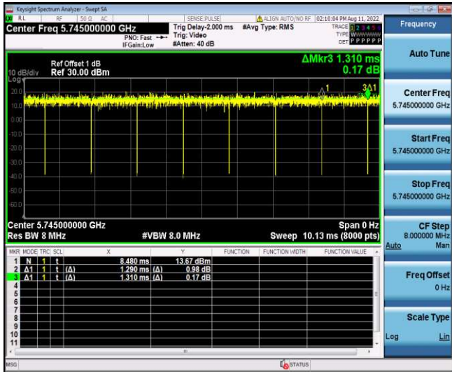
11N20SISO_Ant2_5745
