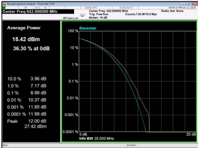
Figure 352: QPSK 20MHz B.W; 642.0MHz, 60kHz
