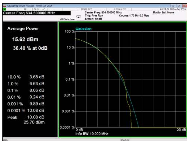
Figure 237: 16QAM 10MHz B.W; 634.5MHz, 30kHz
