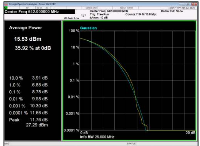
Figure 325: 256QAM 20MHz B.W; 642.0MHz, 60kHz
