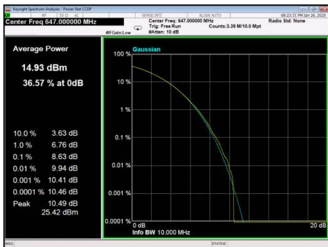
Figure 235: 16QAM 10MHz B.W; 647.0MHz, 15kHz
