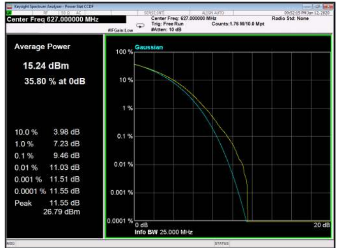
Figure 353: QPSK 20MHz B.W; 627.0MHz, 30kHz
