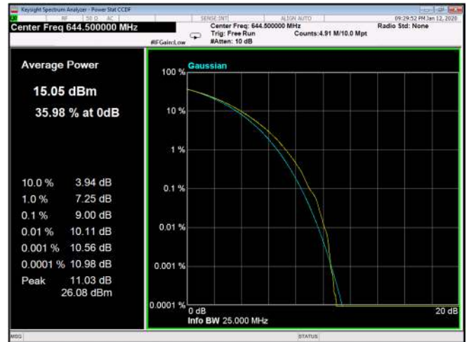
Figure 343: QPSK 15MHz B.W; 644.5MHz, 15kHz
