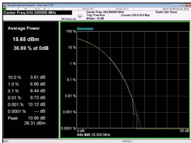
Figure 255: 16QAM 20MHz B.W; 634.5MHz, 30kHz
