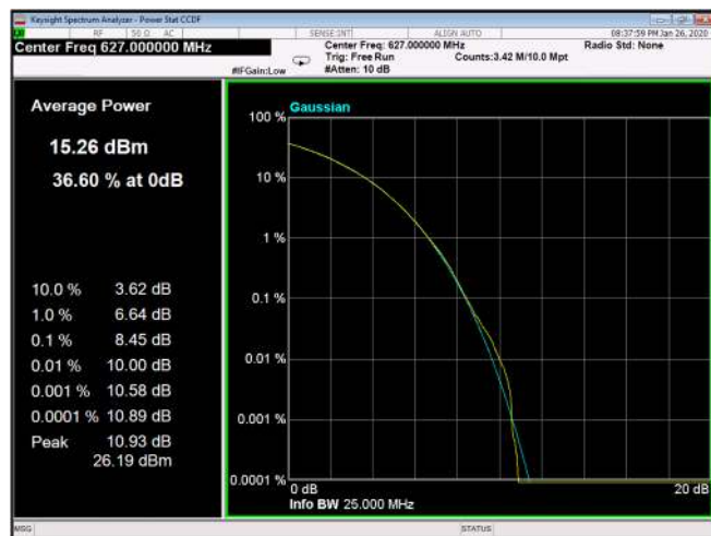
Figure 254: 16QAM 20MHz B.W; 627.0MHz, 30kHz
