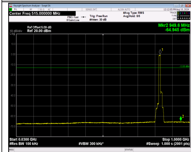
5-5-10MHz-10MHz-QPSK-QPSK-20476-20575-50RB#0-050RB#0-30~1000MHz-PASS
