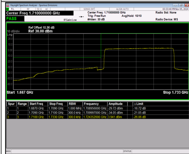
Band4-20MHz-QPSK-20300-1RB#99
