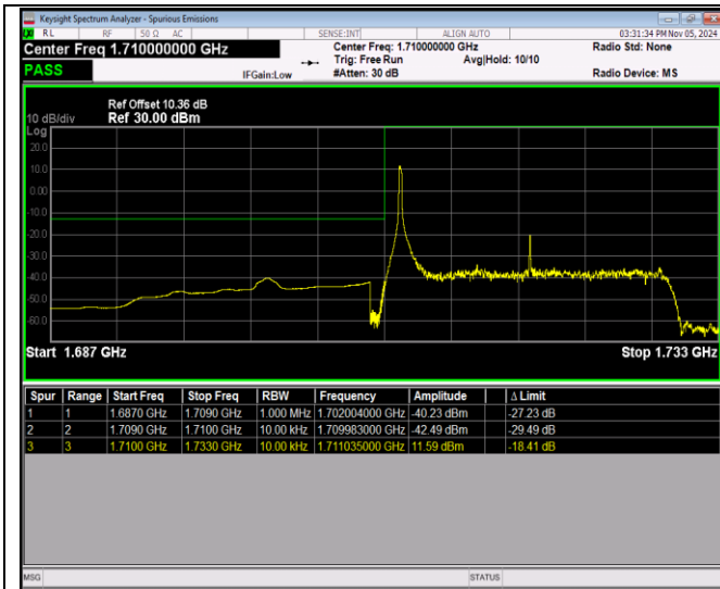
Band4-20MHz-QPSK-20050-100RB#0
