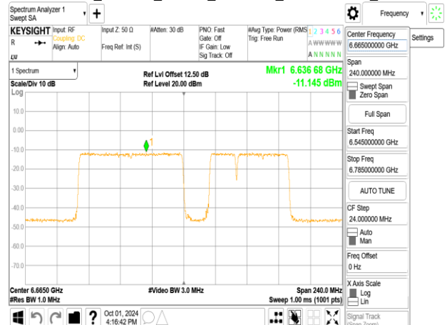
802.11be_160MHz_ChainB_6665MHz_996+484+242_MR05
