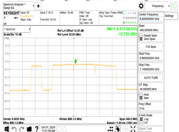
802.11be_320MHz_ChainA_6905MHz_3x996+484_MRU2
