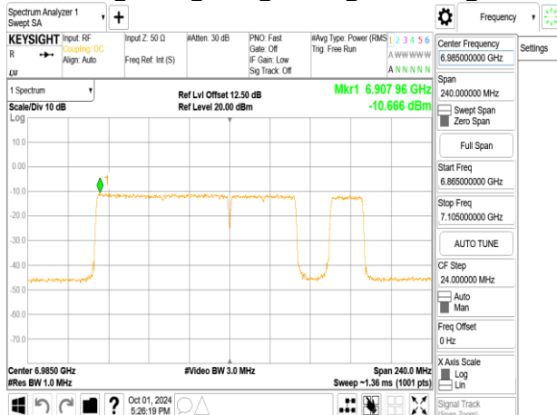
802.11be_160MHz_ChainB_6985MHz_996+484+242_MRU7
