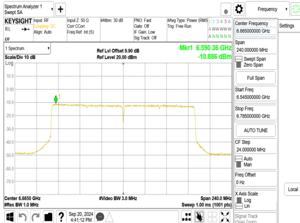
802.11be_160MHz_ChainB_6665MHz_996+484+242_MR01
