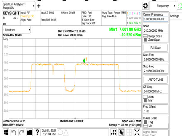
802.11be_160MHz_ChainB_6985MHz_996+484+242_MRU5
