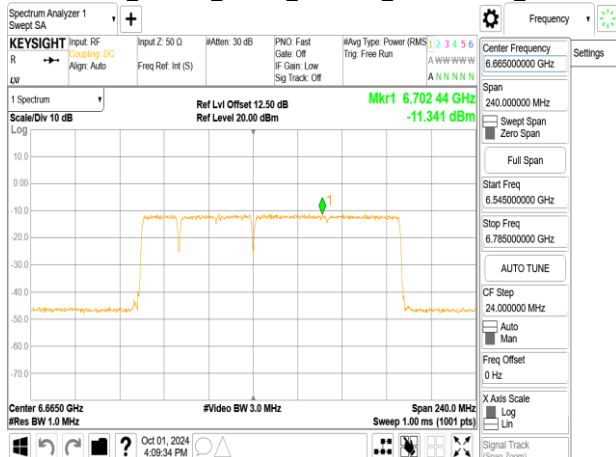
802.11be_160MHz_ChainB_6665MHz_996+484+242_MR01
