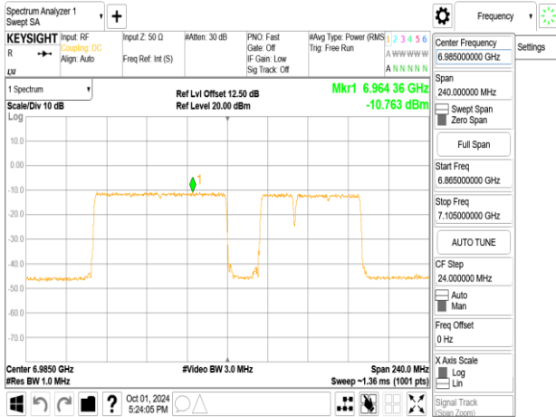
802.11be_160MHz_ChainA_6985MHz_996+484+242_MR07
