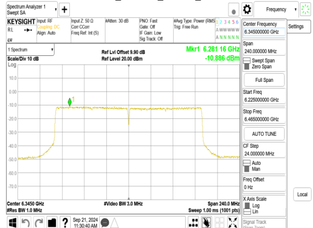
802.11be_160MHz_ChainB_6345MHz
