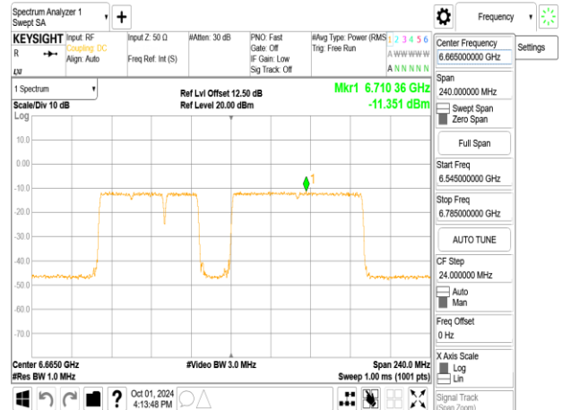
802.11be_160MHz_ChainB_6665MHz_996+484+242_MR05
