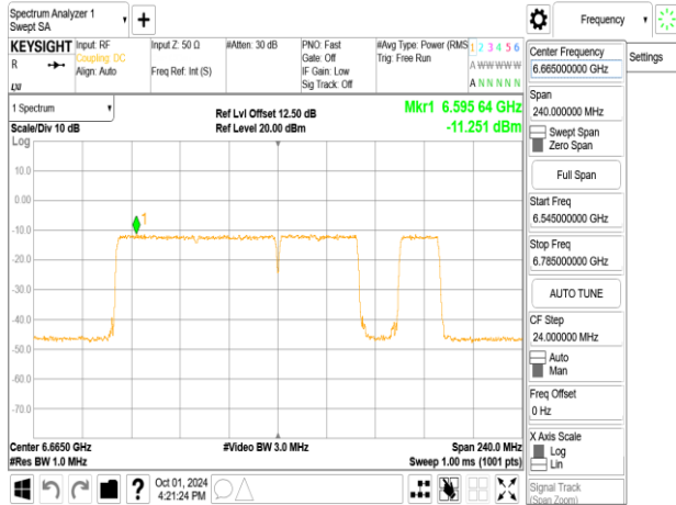
802.11be_160MHz_ChainB_6665MHz_996+484+242_MR08
