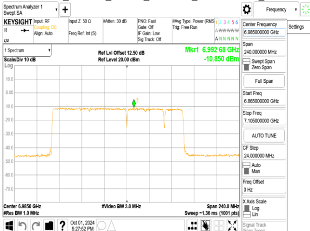
802.11be_160MHz_ChainA_6985MHz_996+484+242_MR08
