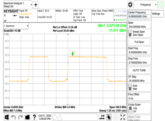
802.11be_160MHz_ChainB_6665MHz_996+484_MR03
