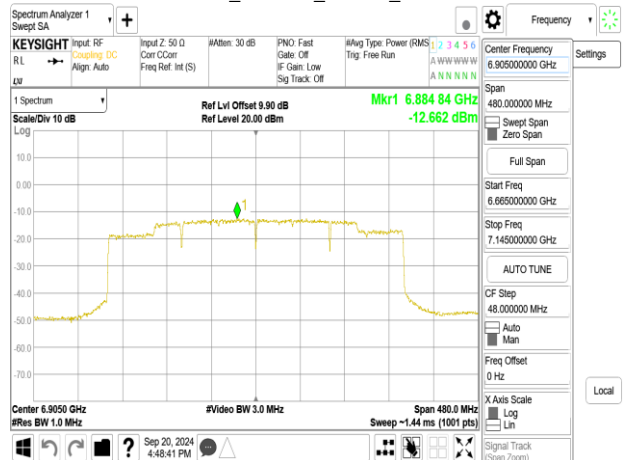
802.11be_320MHz_ChainA_6905MHz_3x996+484_MRU1
