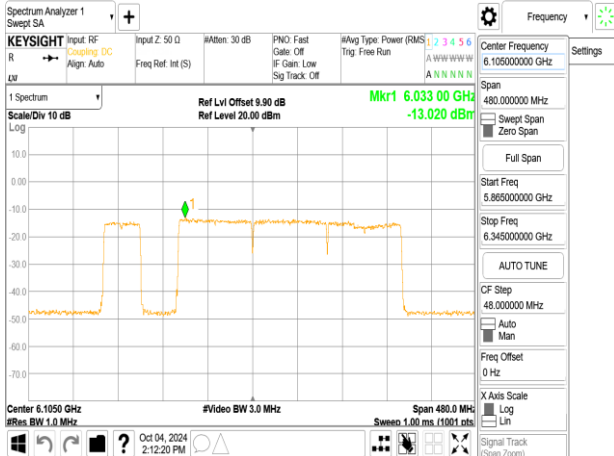
802.11be_320MHz_ChainA_6105MHz_3x996+484_MRU8
