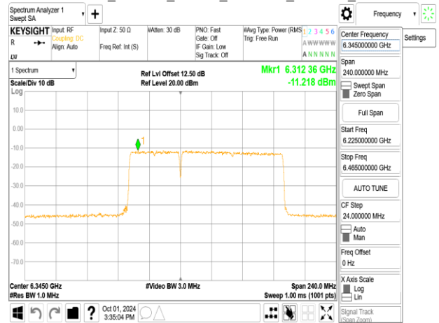
802.11be_160MHz_ChainB_6345MHz_996+484_MR3
