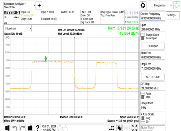
802.11be_160MHz_ChainA_6985MHz_996+484_MR03
