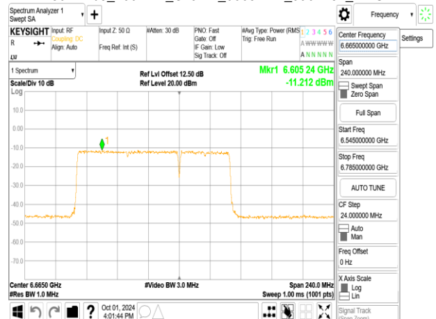
802.11be_160MHz_ChainB_6665MHz_996+484_MR04
