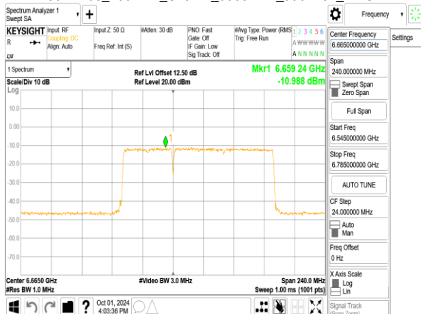
802.11be_160MHz_ChainB_6665MHz_996+484_MR01
