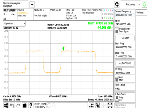
802.11be_160MHz_ChainB_6985MHz_996+484_MRU2
