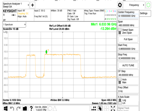
802.11be_320MHz_ChainA_6105MHz_2x996+484_MRU2
