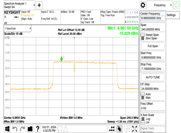
802.11be_160MHz_ChainA_6985MHz_996+484_MR02
