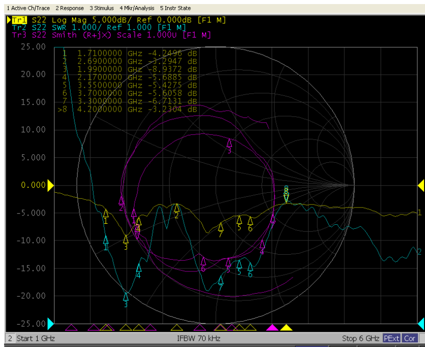
ANT4
