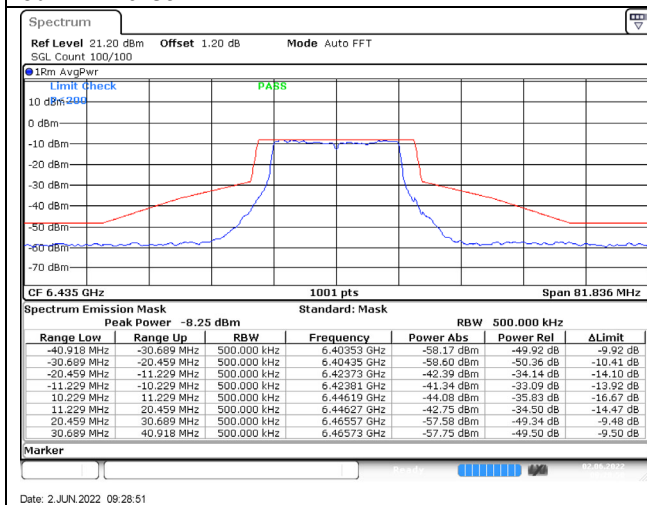
802.11a / 6435MHz / Chain C / NSS-4
