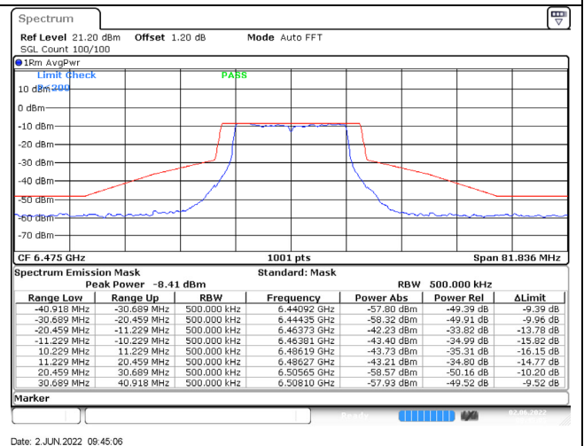
802.11a / 6475MHz / Chain B / NSS-4
