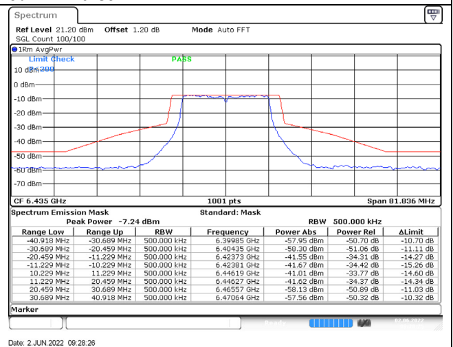
802.11a / 6435MHz / Chain D / NSS-4
