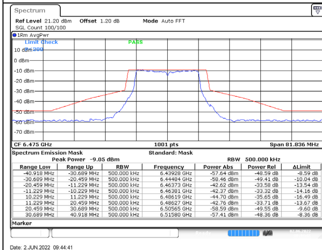
802.11a / 6475MHz / Chain A / NSS-4
