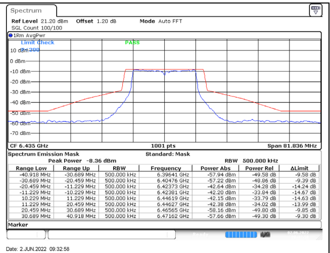
802.11a / 6435MHz / Chain B / NSS-4
