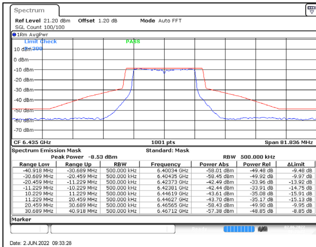
802.11a / 6435MHz / Chain A / NSS-4
