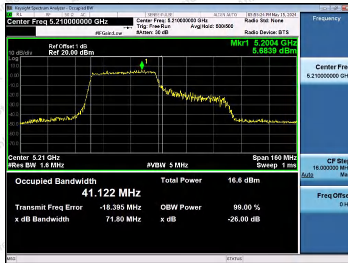
11AX80SISO-Ant1-5210-484Tone-RU65
