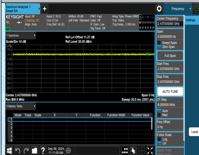
NTNV-11N20MIMO-Ant3-2437
