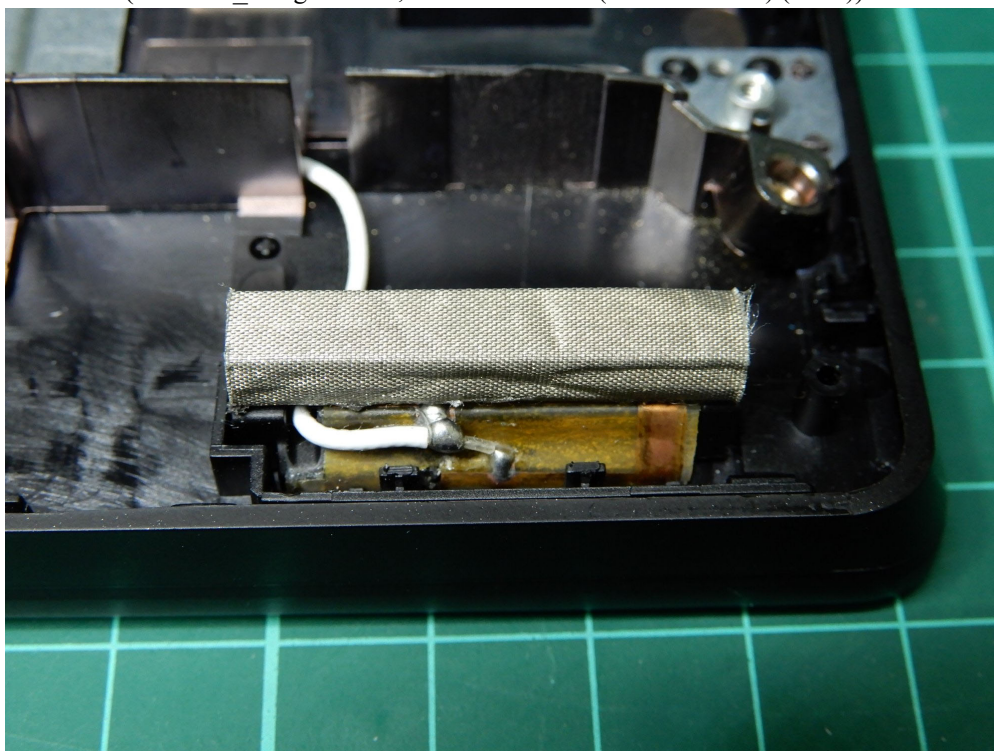
(56) EUT Photo (Antenna_Hong-BO Co., Ltd. / 260-24363 (DC33002IL0L) (Main))
