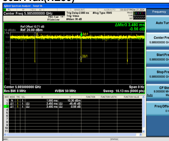
802.11ax(HE80)
