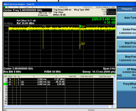
802.11ax(HE40)
