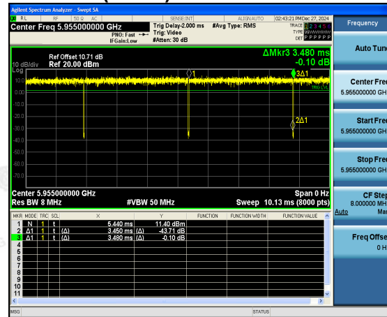
802.11ax(HE20)
