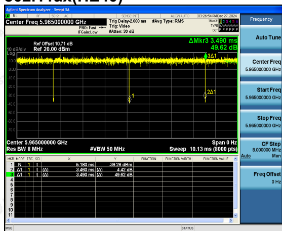
802.11ax(HE40)
