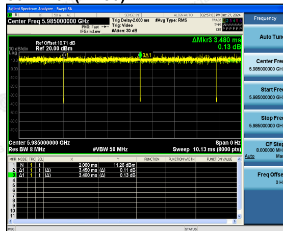
802.11ax(HE80)
