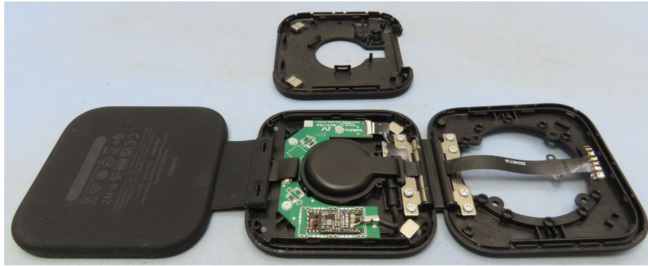
Mainboard 1 PCBA
