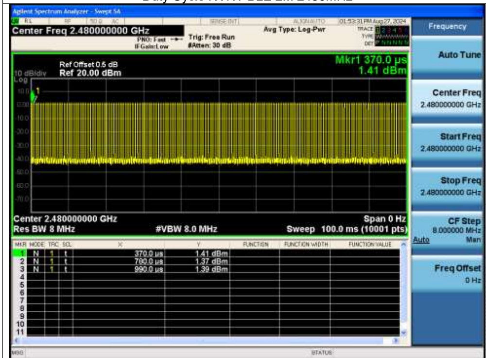
Duty Cycle NVNT BLE 2M 2480MHz
