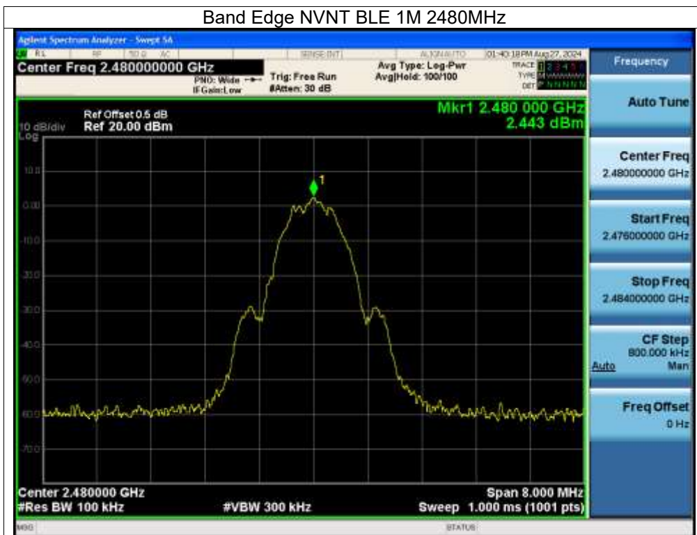
Band Edge NVNT BLE 1M 2480MHz Emission
