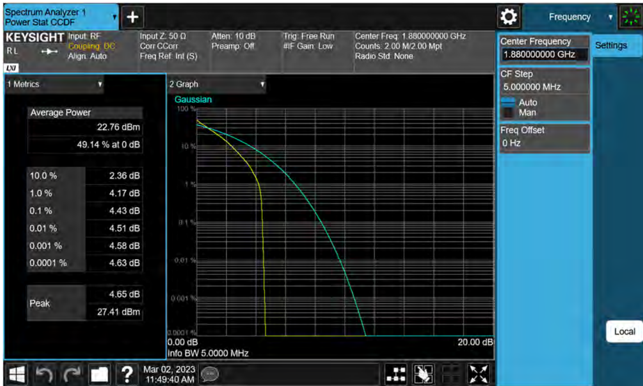
Sub6 n2. PAR Plot (5 M BW Ch.376000 QPSK RB 25_0)
