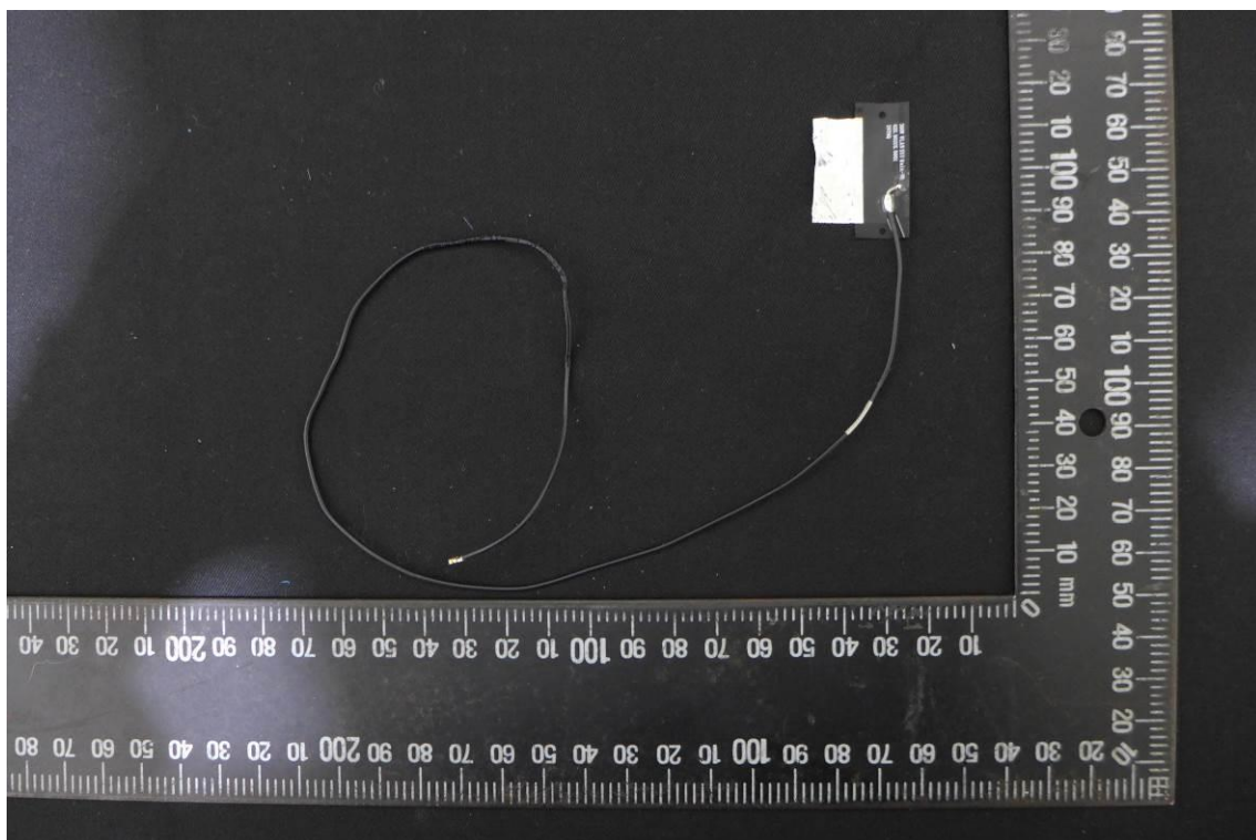
Antenna: INPAQ/025.901U5.0001
