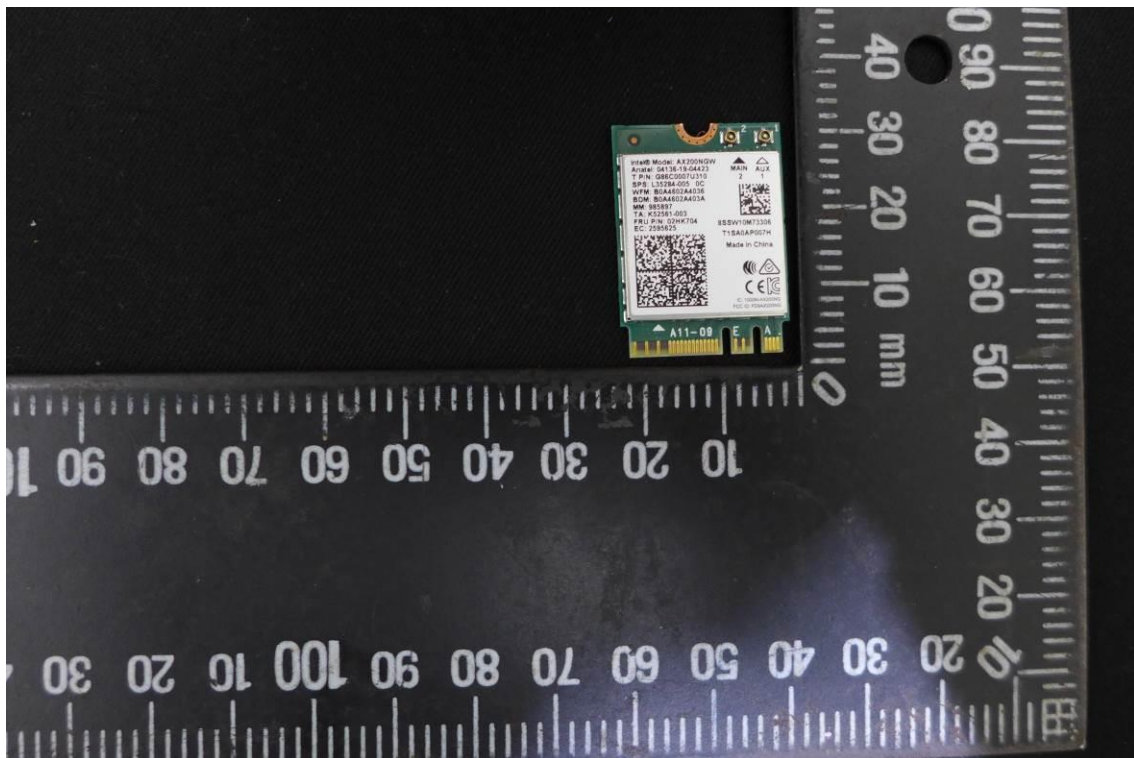
Module: AX200NGW
