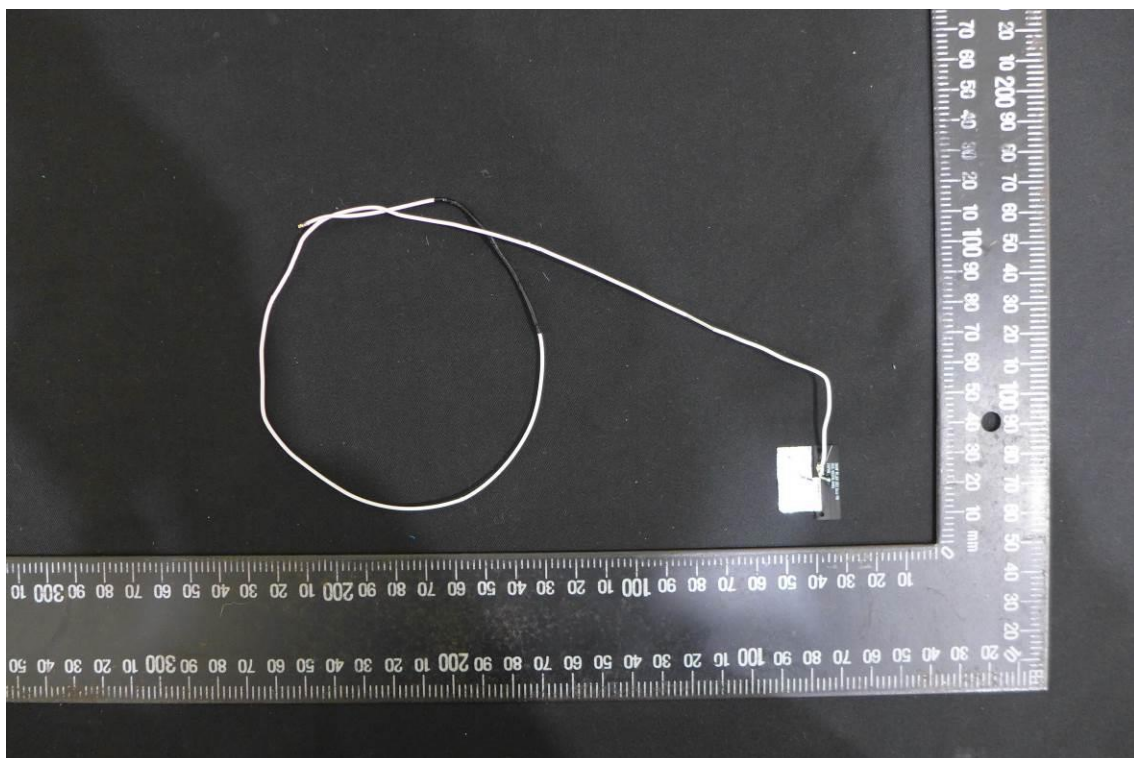
Antenna: INPAQ/025.901U6.0001
