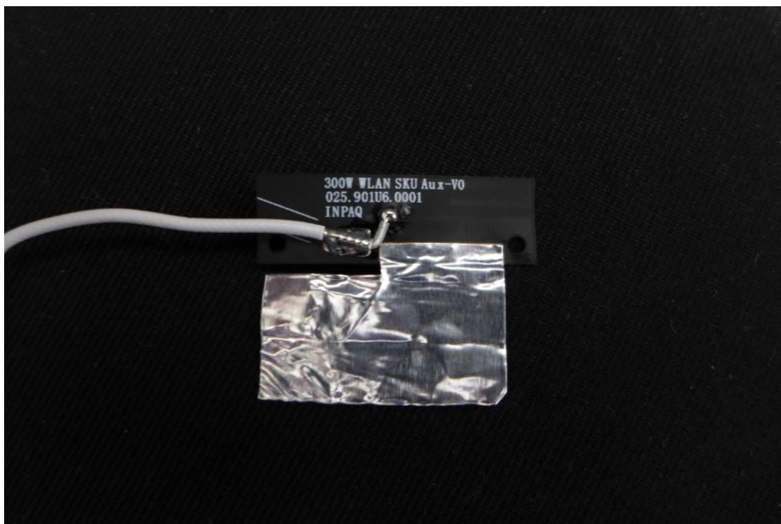
Antenna: INPAQ/025.901U6.0001
