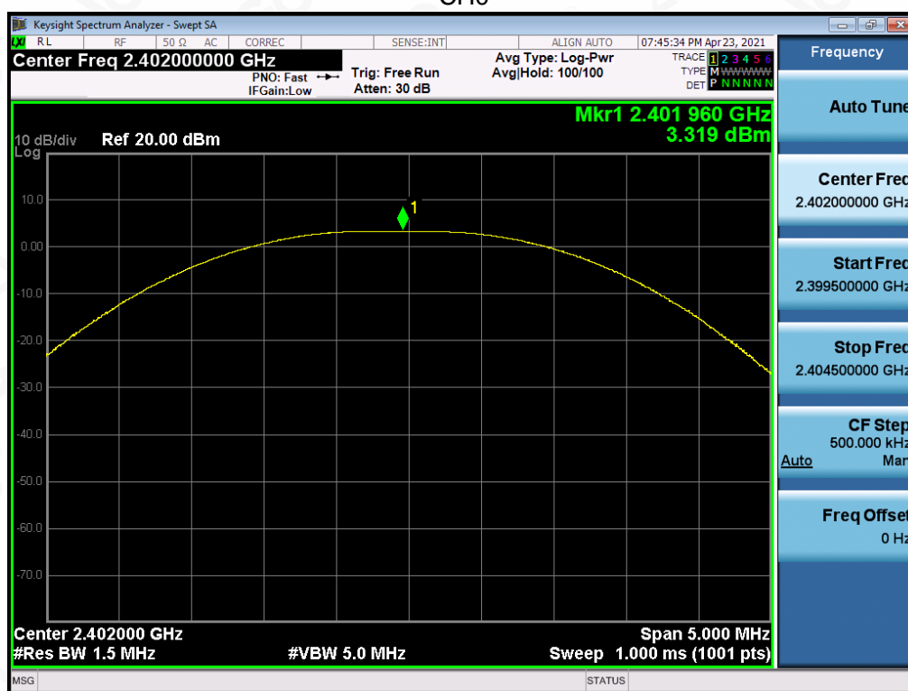
\text{CHO}
