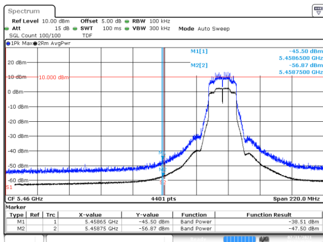
BE-R-LOW, MIMO-A, 802.11ax20-HE0, Ch100
