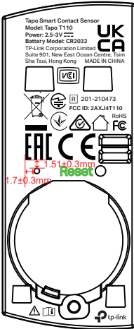
尺寸图
