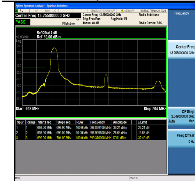
Band12 5MHz 64QAM 23035 1RB#0
