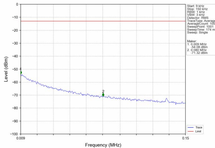
Band2_20MHz_16QAM_HCH_1900MHz_RB_1_0_NTNV
