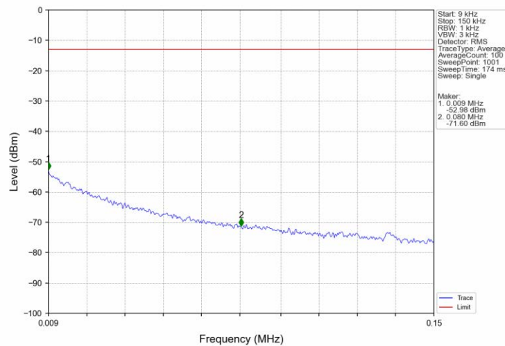
Band2_10MHz_16QAM_HCH_1905MHz_RB_1_0_NTNV
