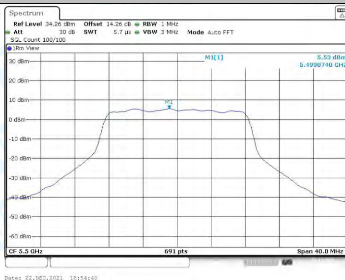
11A_Ant3_5500
