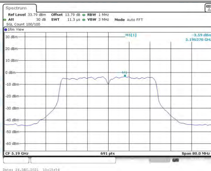
11N40MIMO_Ant3_5190
