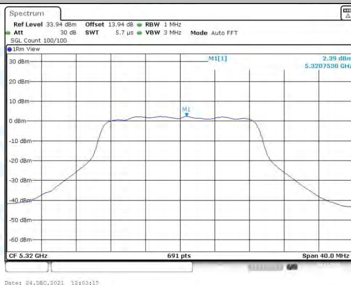
11AC20MIMO_Ant3_5320
