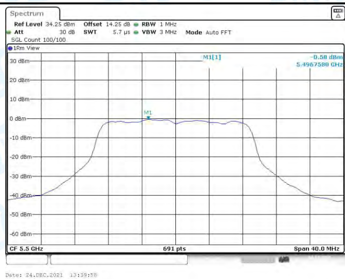
11AC20MIMO_Ant1_5500
