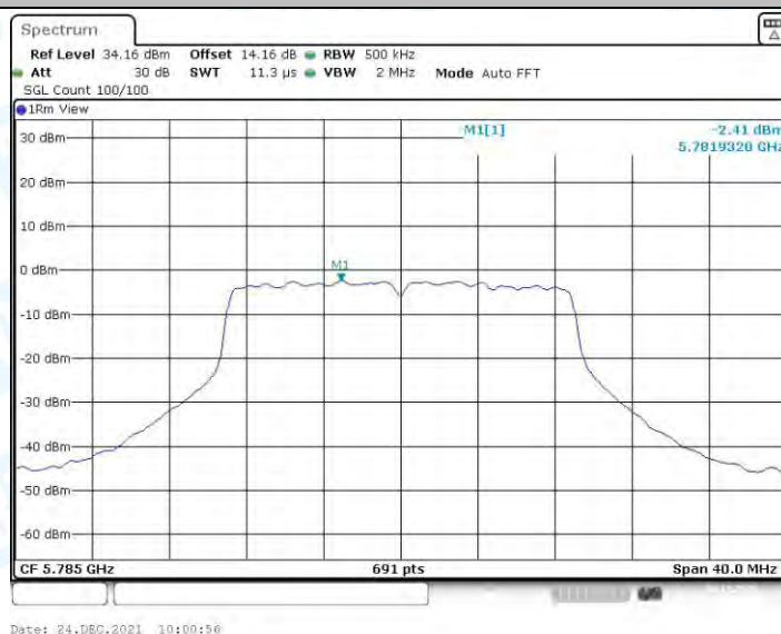
11N20MIMO_Ant3_5785
