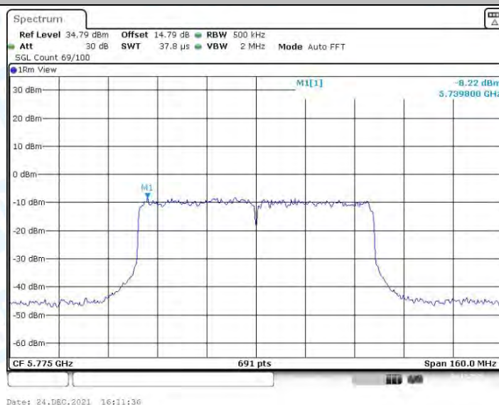
11AC80MIMO_Ant3_5775
