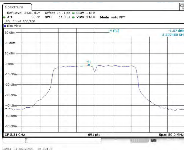
11N40MIMO_Ant3_5310
