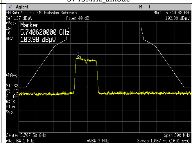
5755MHz_n40mode
