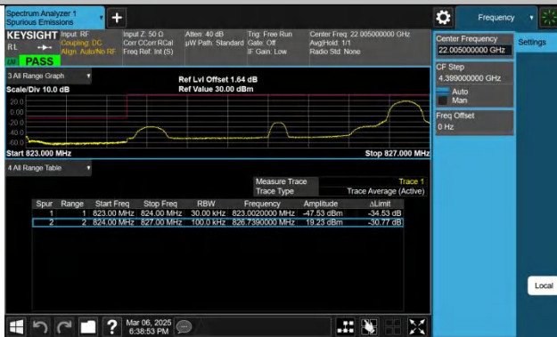
Band26(824-849)-3MHz-QPSK-26805-1RB#14-PASS
