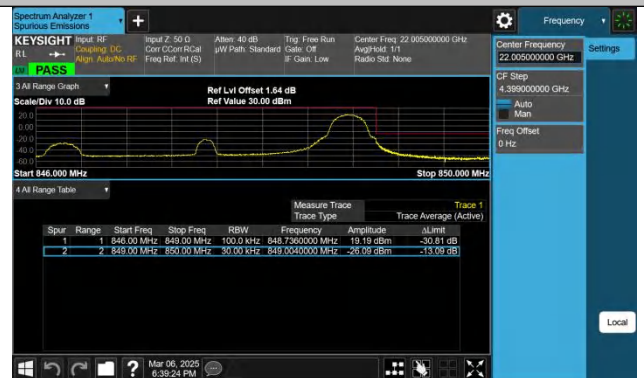
Band26(824-849)-3MHz-QPSK-27025-1RB#14-PASS
