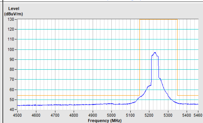
Vertical (Average)
