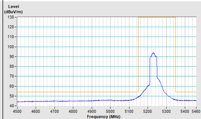
Horizontal (Average)
