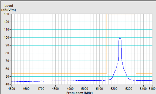
Vertical (Average)
