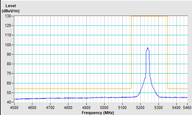
Horizontal (Average)
