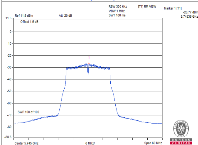
802.11n (HT20) : CH 149
