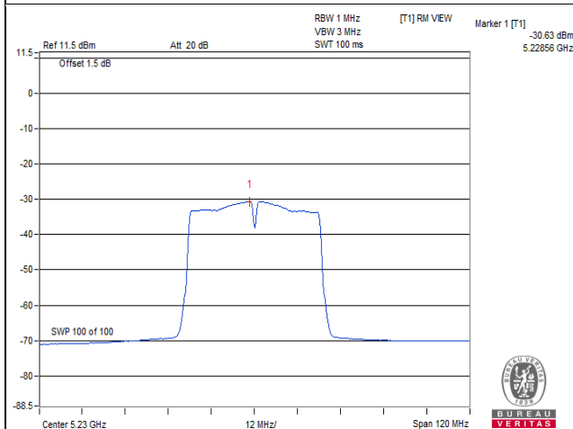
802.11n (HT40) : CH 46
