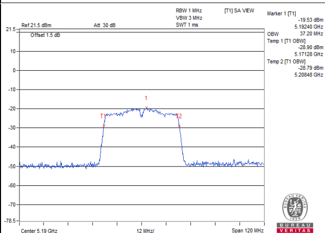
802.11n (HT40) : CH 38
