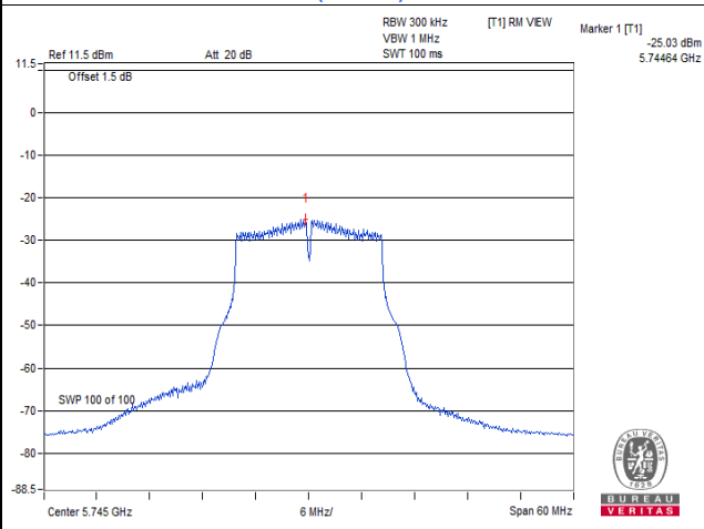
802.11a : CH 149
