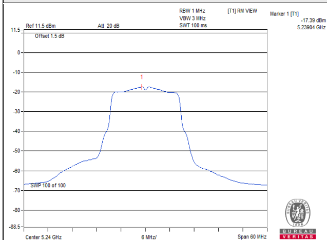
802.11a : CH 48
