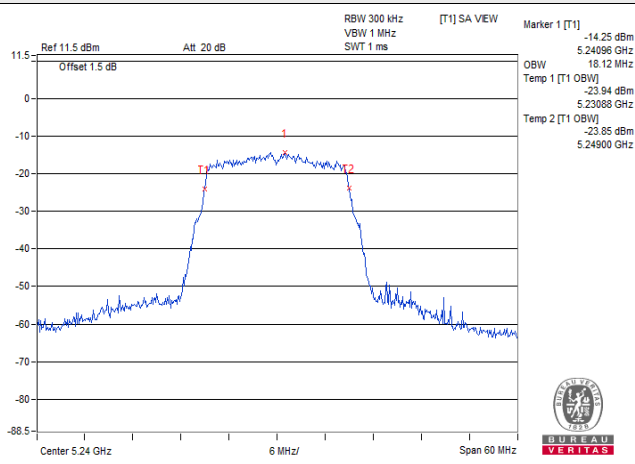
802.11n (HT20) : CH 48
