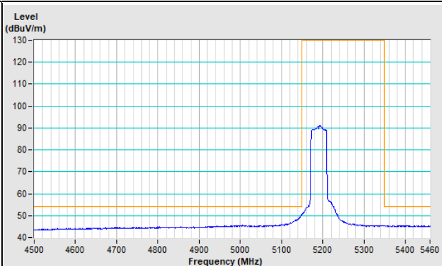
Horizontal (Average)
