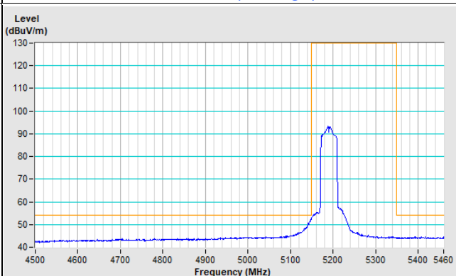
Vertical (Average)
