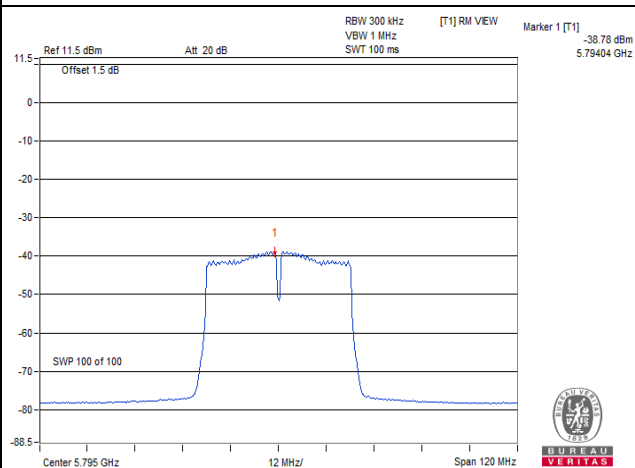
802.11n (HT40) : CH 159
