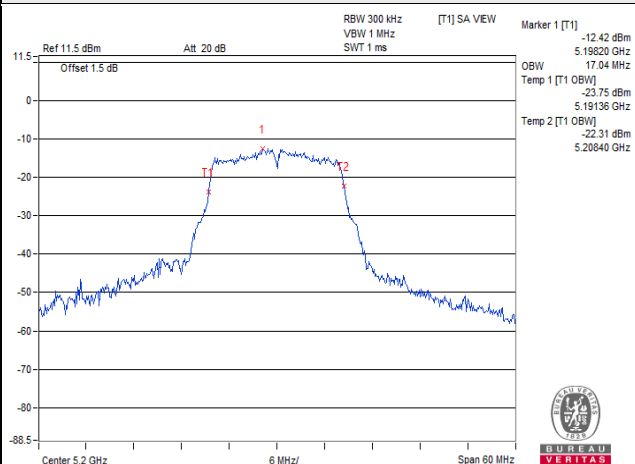
802.11a : CH 40
