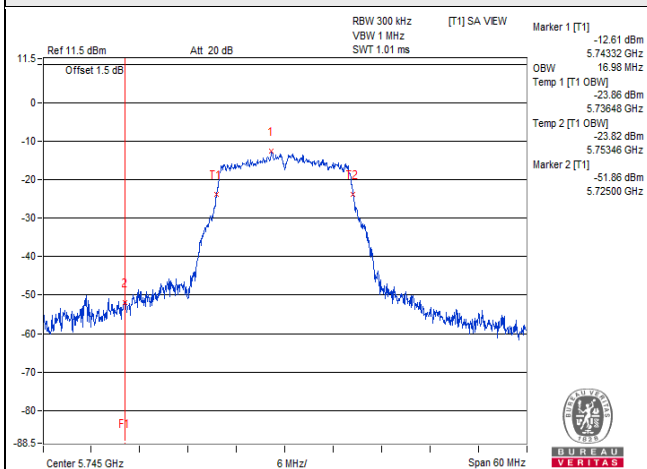
802.11a : CH 149
