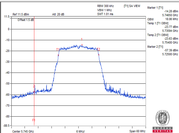
802.11n (HT20) : CH 149
